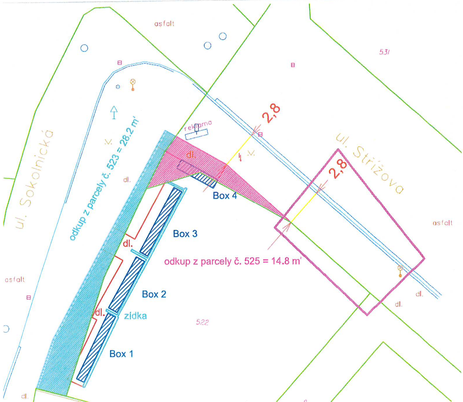
geometrický plán č.2
