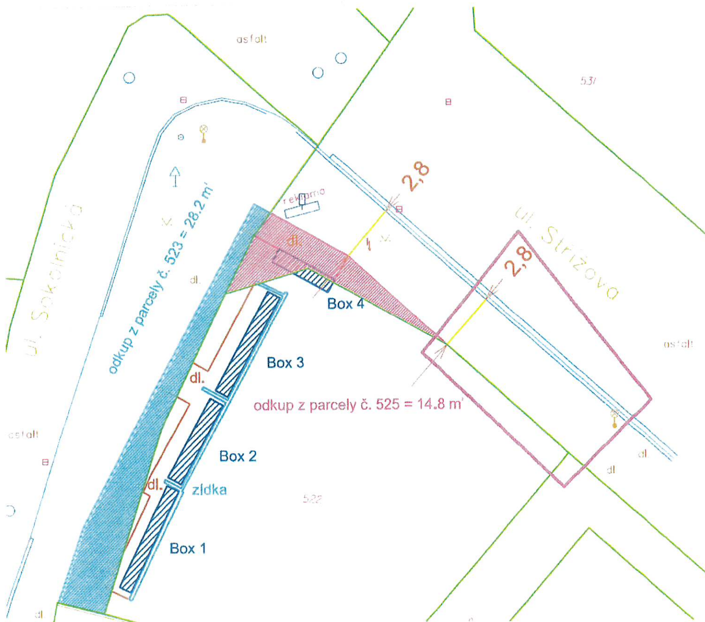
geometrický plán č.2
